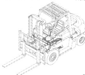
行车制动管路系统 BRAKE PIPING SYSTEM
