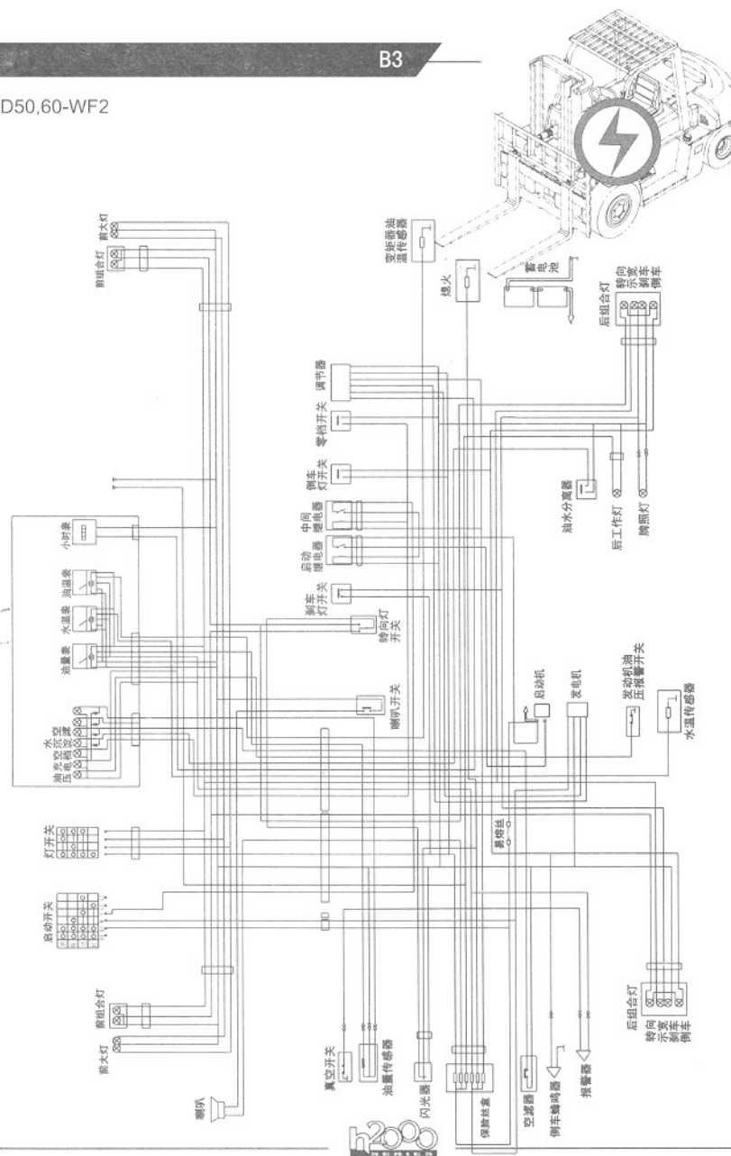
电气系统/ELECTRIC SYSTEM
