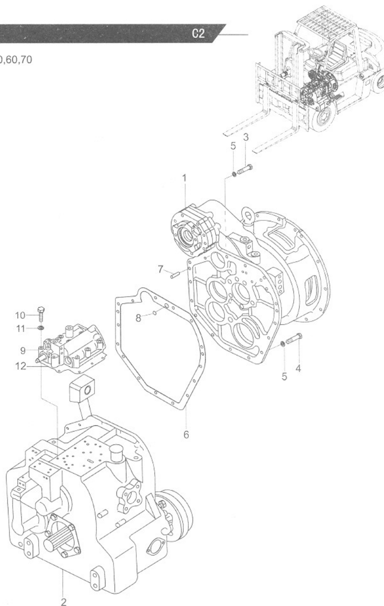
传动装置/DRIVE UNIT
